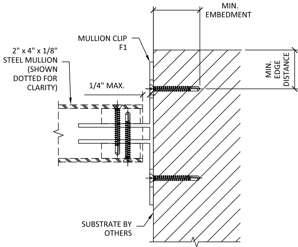
A 3 VERTICAL SECTION CLIP F1 INSTALLATION
